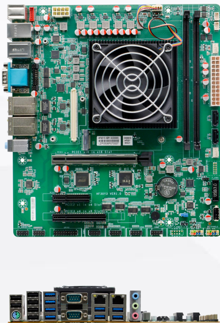
接口标示图：
