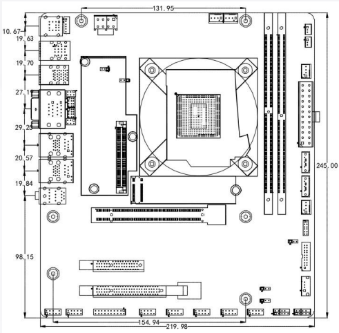
产品尺寸图：
